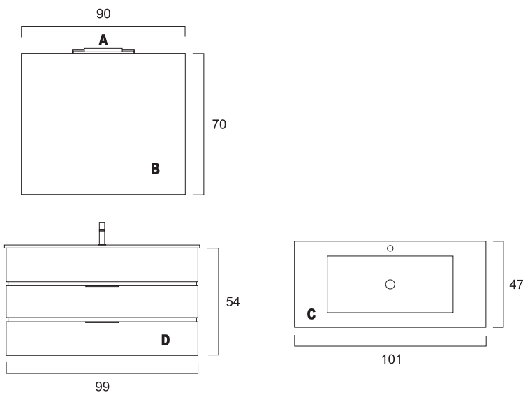
Vista de Frente Prof. máxima móvel: 45 Vista de Cima do Tampo de Vidro
