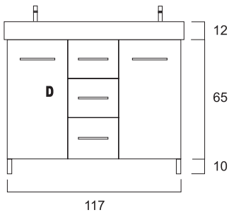
Vista de Frente Prof. máxima móvel: 47
