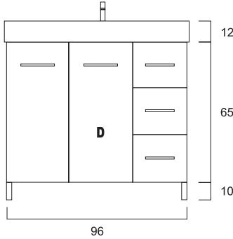
Vista de Frente Prof. máxima móvel: 47
