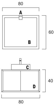
Vista de Frente Prof. máxima móvel: 45
