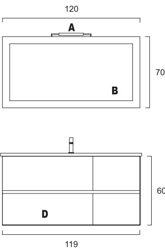
Vista de Frente Prof. máxima móvel: 45
