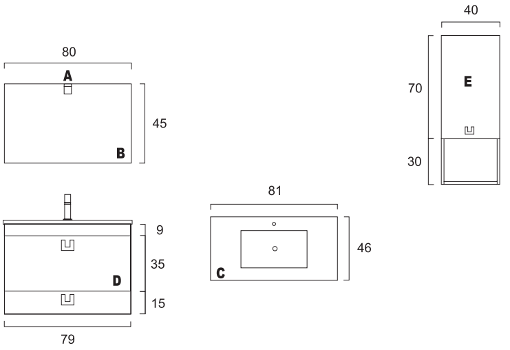
Vista de Frente Prof. máxima móvel: 45 Vista de Cima do Lavatório Vista de Frente Prof. máxima coluna: 25
