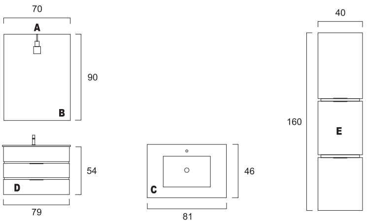
Vista de Frente Prof. máxima móvel: 45 Vista de Cima do Lavatório Prof. máxima coluna: 25
