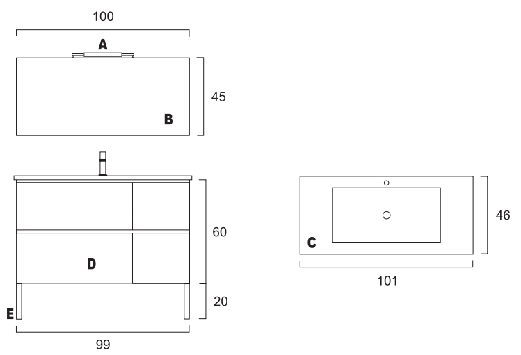
Vista de Frente Prof. máxima móvel: 45 Vista de Cima do Lavatório
