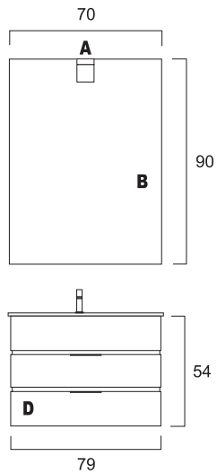
Vista de Frente Prof. máxima móvel: 45
