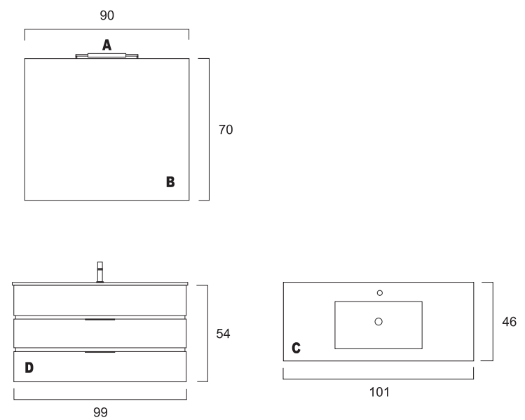
Vista de Frente Prof. máxima móvel: 45 Vista de Cima do Lavatório
