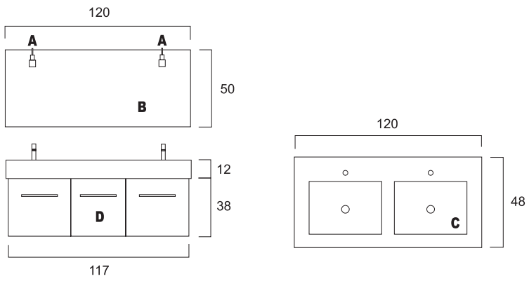
Vista de Frente Prof. máxima móvel: 47
