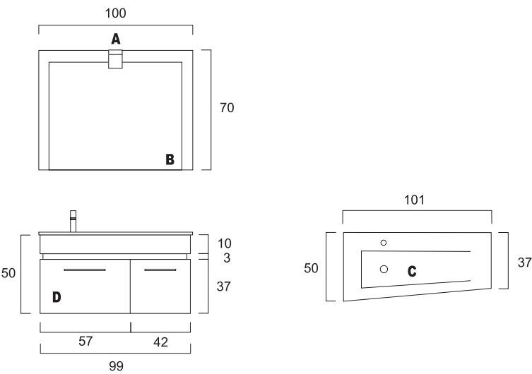
Vista de Frente Prof. máxima móvel: 49
