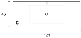
Vista de Cima do Lavatório
