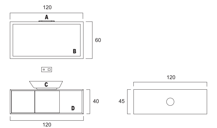
Vista de Frente Prof. máxima móvel: 45
