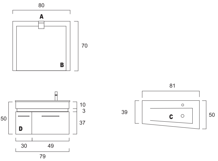
Vista de Frente Prof. máxima móvel: 49 Vista de Cima do Lavatório
