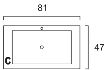
Vista de Cima do Tampo de Vidro
