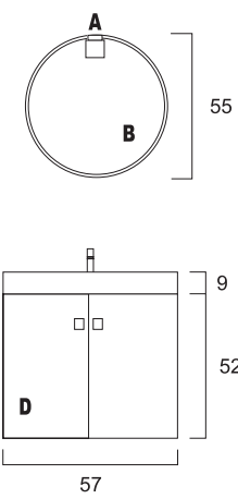
Vista de Frente Prof. máxima móvel: 43
