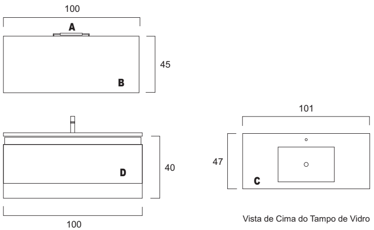
Vista de Frente Prof. máxima móvel: 46
