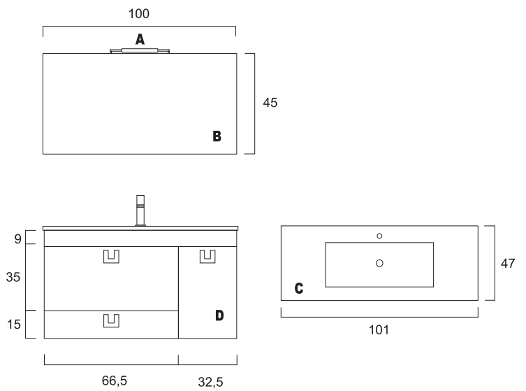
Vista de Frente Prof. máxima móvel: 45
