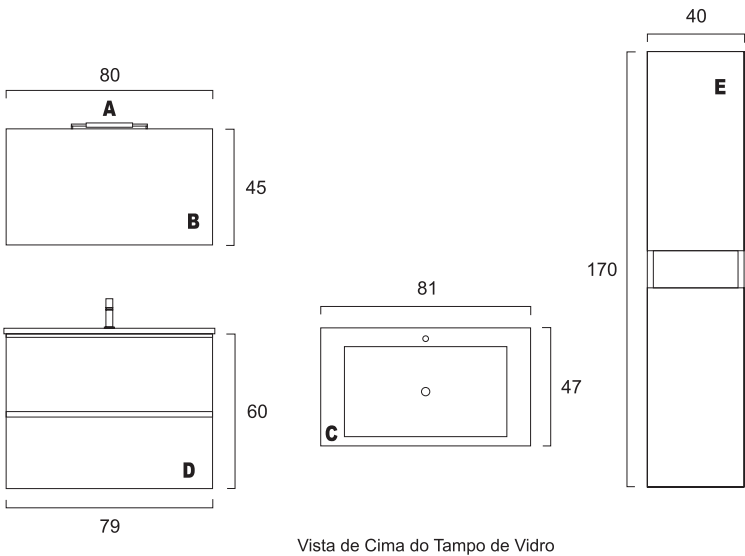
Vista de Frente Prof. máxima móvel: 45 Vista de Frente Prof. máxima coluna: 25
