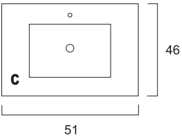
Vista de Cima do Lavatório
