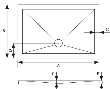
POSIÇÃO DA VÁLVULA AO CENTRO (1)
